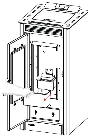
EXTRACCION CENIZERO PARA LIMPIEZA
