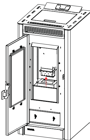
EXTRACCION QUEMADOR PARA LIMPIEZA
