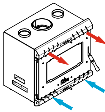
Circulación hacia el ambiente
