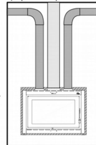
Ejemplo de salida por los laterales
