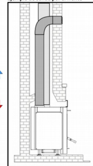
Ejemplo de salida por el frente
